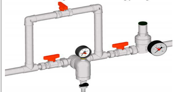
Установка на горизонтальном трубопроводе
