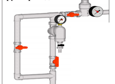
Установка на вертикальном трубопроводе
